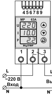
Схема подключения
